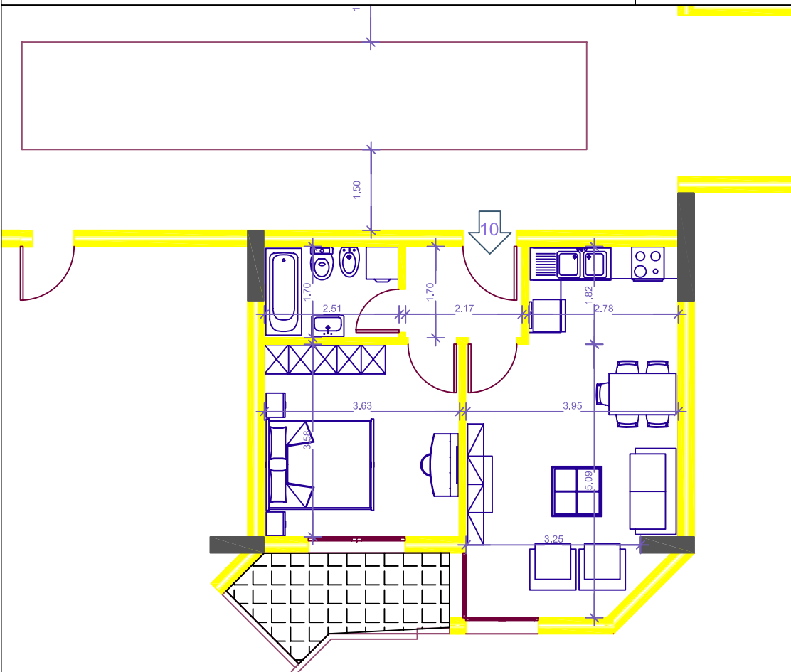
PLANIMETRIA E APARTAMENTIT 10 / KT PESTE SH 1: 100 ( OBJEKTI 2 )
