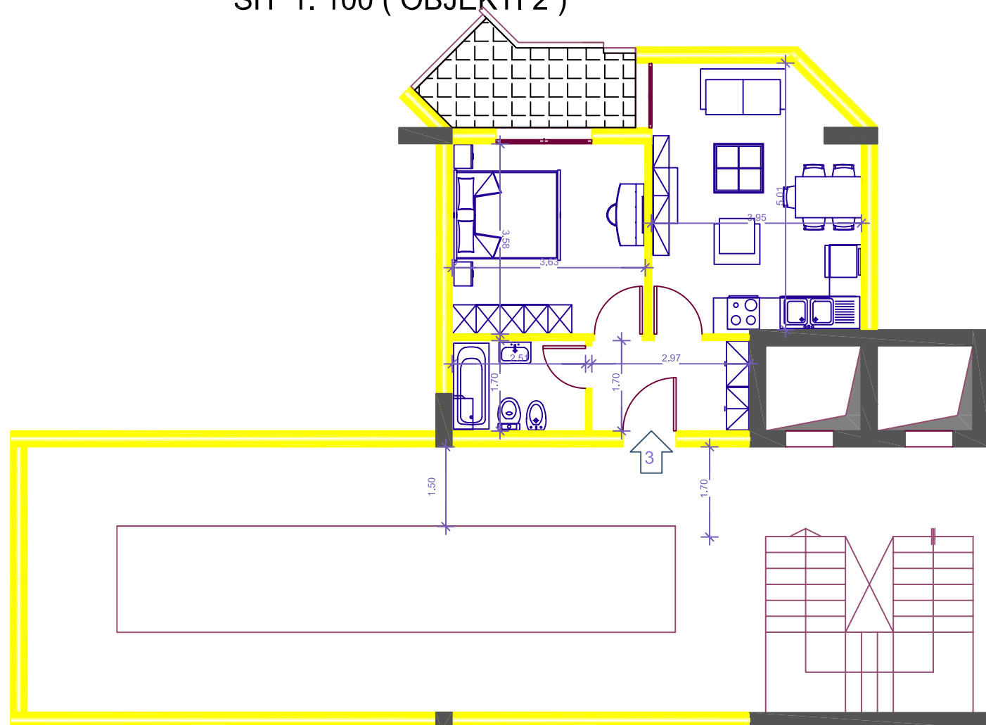
PLANIMETRIA E APARTAMENTIT 3 / KT PESTE SH 1: 100 ( OBJEKTI 2 )
