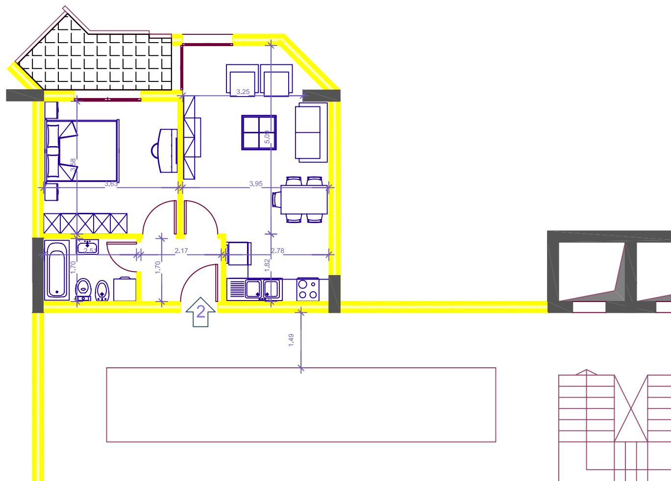
PLANIMETRIA E APARTAMENTIT 2/KT PESTE SH 1: 100 (OBJEKTI 2)
