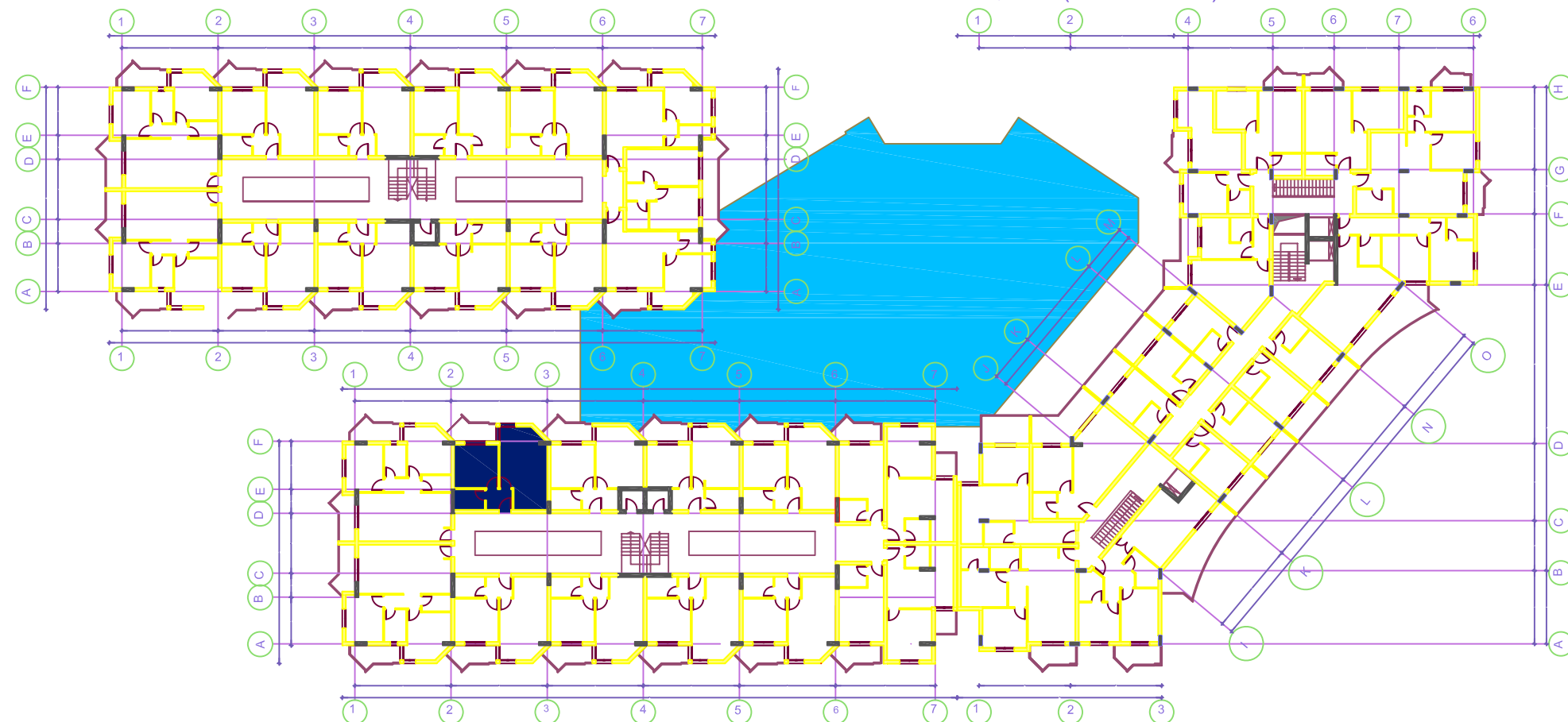
PLANI I VENDOSJES SH 1 : 500 2 , kt 5 (OBJEKTI 2 )
