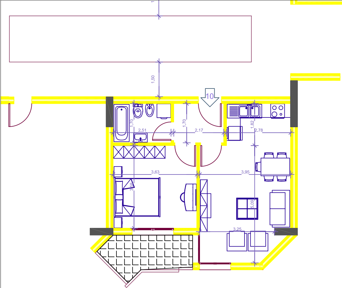
PLANIMETRIA E APARTAMENTIT 10 / KT TRETE SH 1: 100 ( OBJEKTI 2 )
